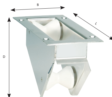
Art. nr.: 10920 Plattformrulle 217 mm nedfelt – D: 250 - B: 116 - L: 216
